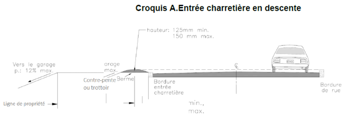
Figure 19 – Démonstration d'une entrée charretière en descente
