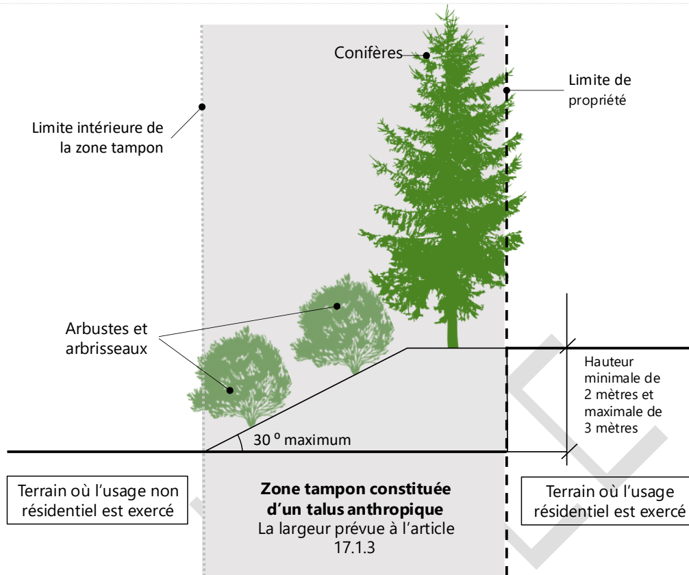
Figure 45 -Zone tampon constituée d'un talus anthropique
