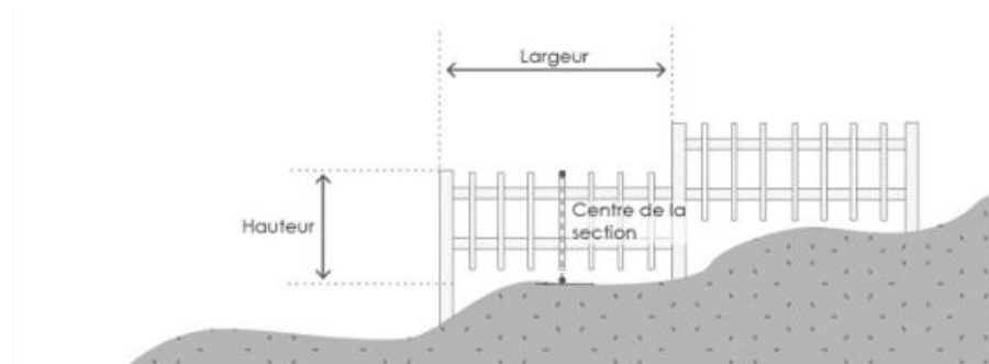
Figure 37 – Hauteur d'une clôture
