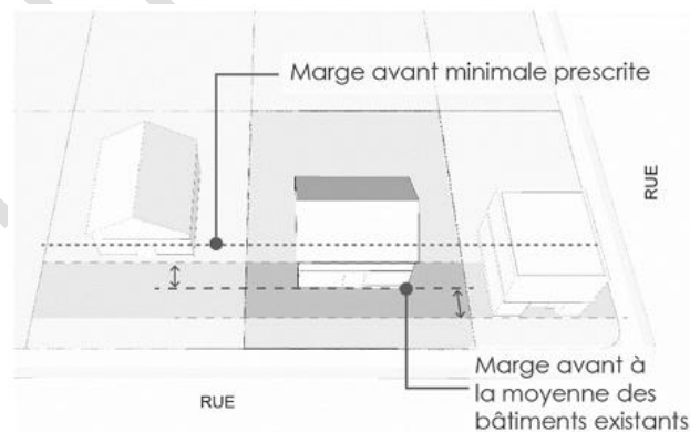
Figure 12 - Marge avant à la moyenne des bâtiments existants dérogoire à la marge prescrite
