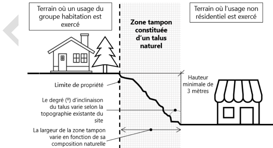
Figure 43 -Zone tampon constituée d'un talus naturel
