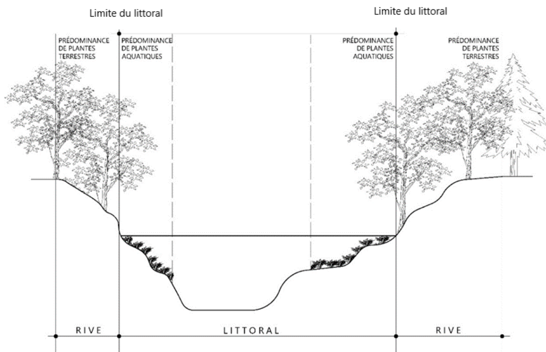
Figure 39 - Délimitation du littoral et de la rive
