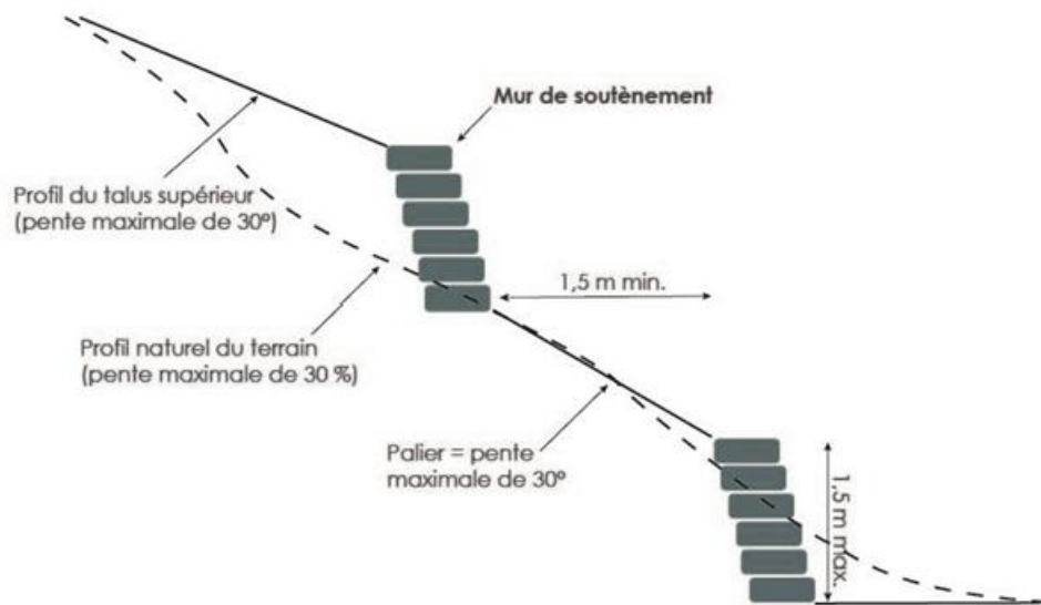
Figure 34 – Construction d'un mur de soutènement
