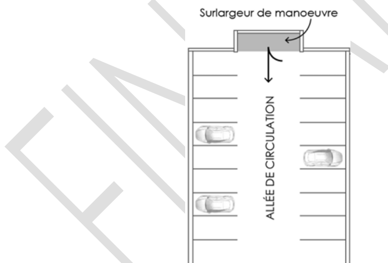
Figure 17 – Démonstration d'une surlargeur de manœuvre
