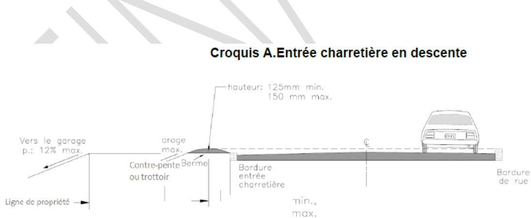
Figure 19 – Démonstration d'une entrée charretière en descente
