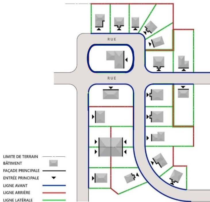
Figure 4 – Désignation des lignes de lot
