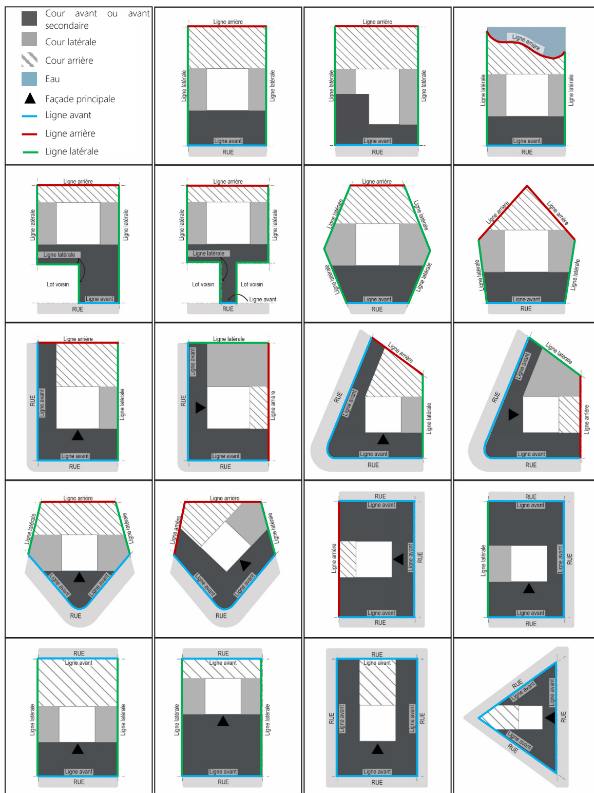
Figure 2 – Schéma d'interprétation des cours
