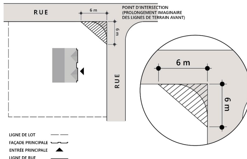
Figure 33 - Schématisation du triangle de visibilité
