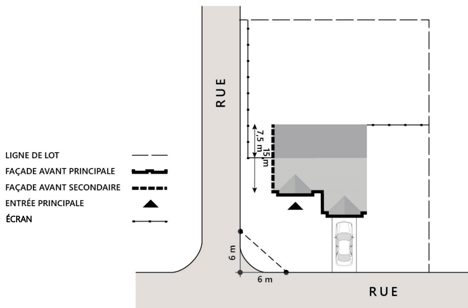
Figure 38 - Démonstration de l'implantation d'un écran d'intimité dans le cas d'un terrain d'angle
