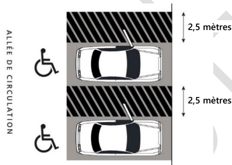
Figure 14 - Schéma d'une bande latérale d'accès pour case de stationnement pour personne à mobilité réduite
