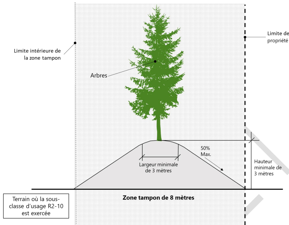
Figure 50 - Zone de mitigation sonore constituée d'une butte-écran végétalisée
