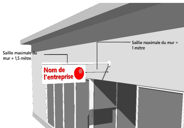
Figure 25 – Démonstration de la saillie maximale pour une enseigne en projection ou perpendiculaire
