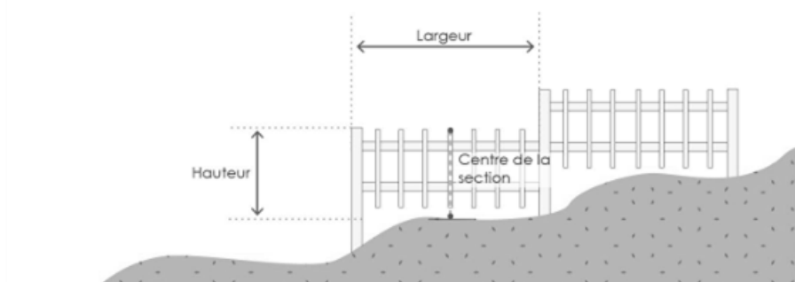
Figure 37 – Hauteur d'une clôture
