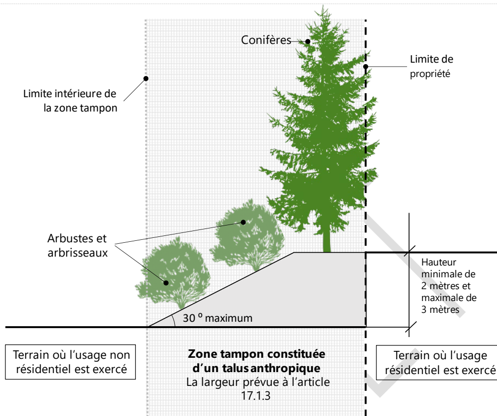
Figure 45 - Zone tampon constituée d'un talus anthropique
