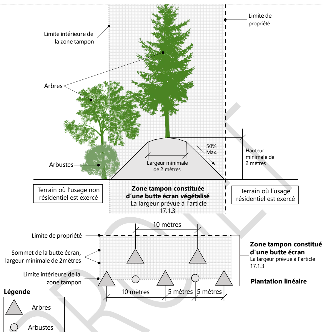
Figure 44 - Zone tampon constituée d'une butte-écran végétalisée
