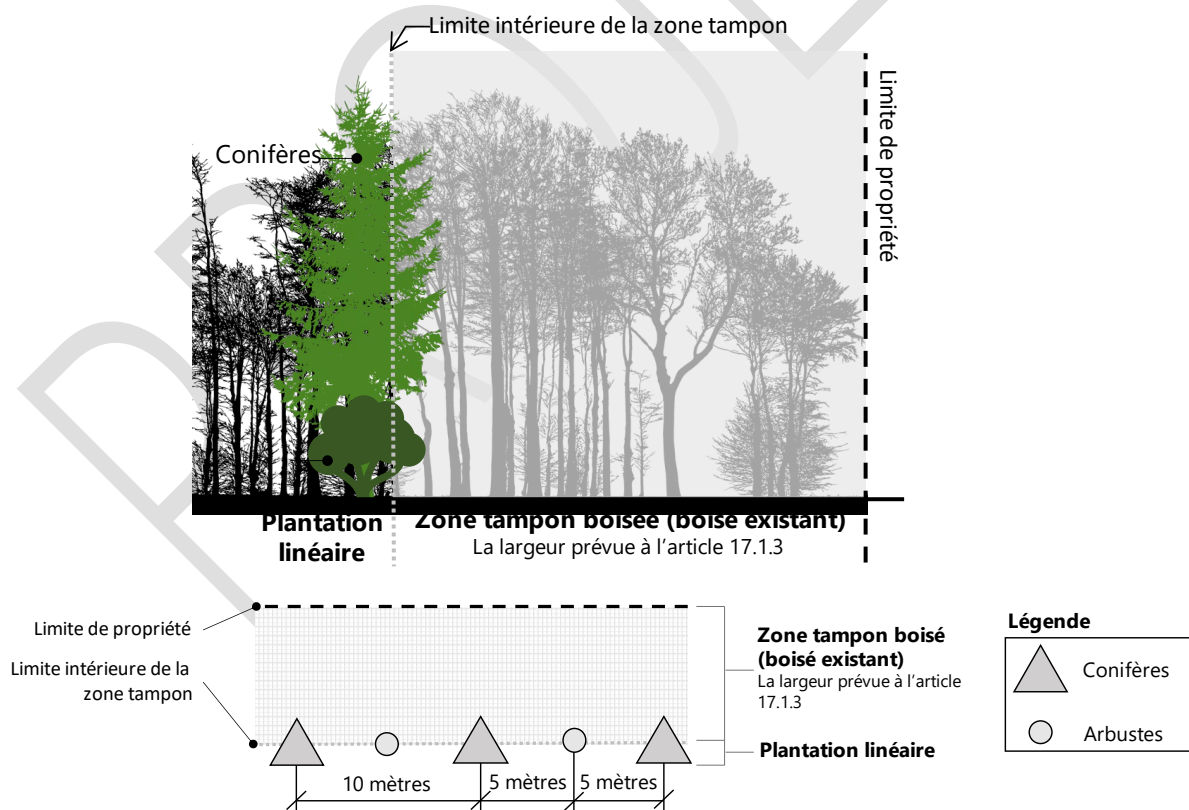
Figure 42 -Zone tampon constituée d'un boisé existant
