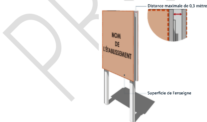
Figure 23 : Démonstration du calcul de la superficie d'une enseigne visible sur les deux côtés
