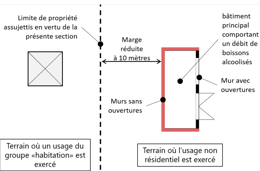
Figure 48 - Profondeur d'une marge relative à un bâtiment principal comportant un débit de boisson alcoolisées.
