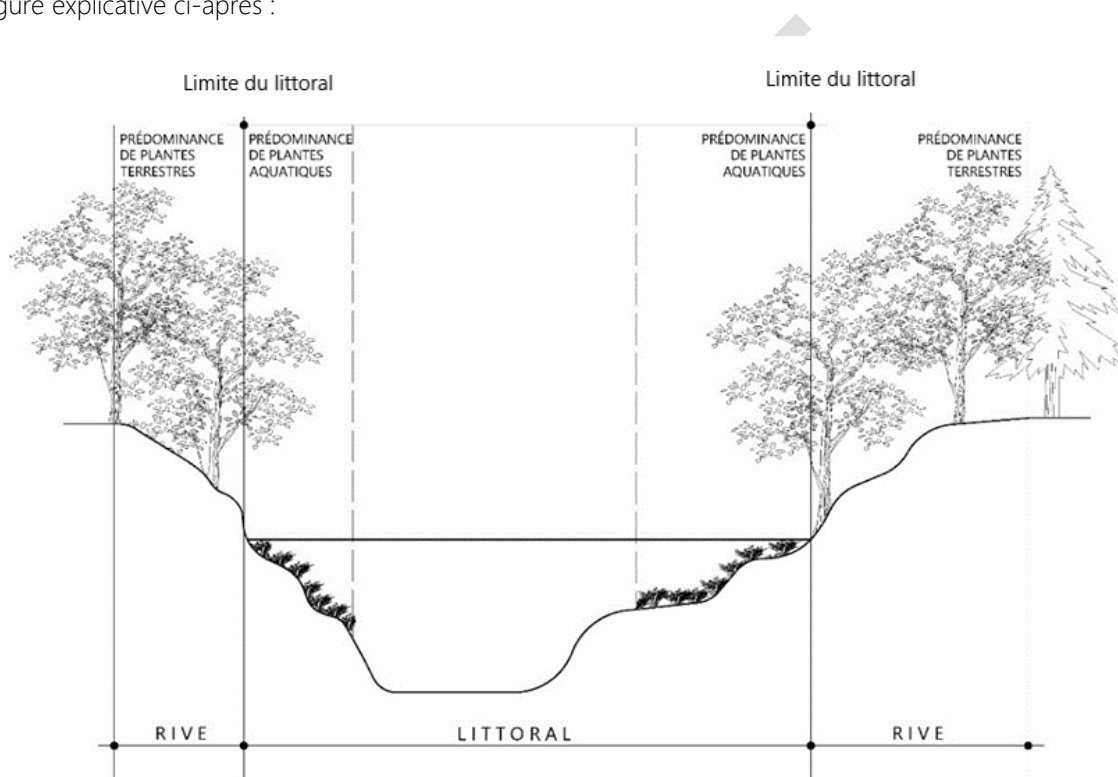
Figure 39 - Délimitation du littoral et de la rive
