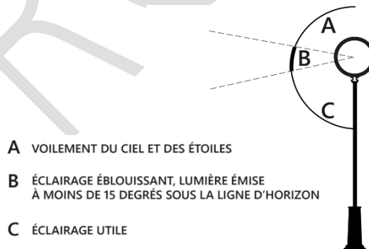
Figure 13 – Représentation des zones d'éclairage
