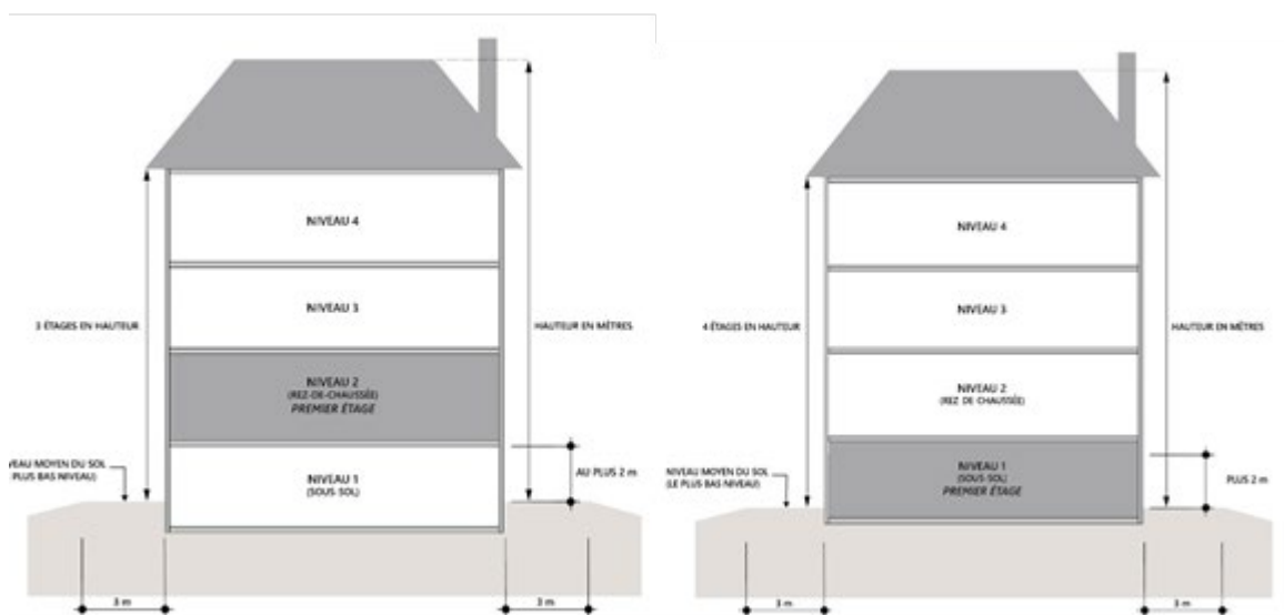
Figure 10 - Démonstration du calcul du nombre d'étages d'un bâtiment
