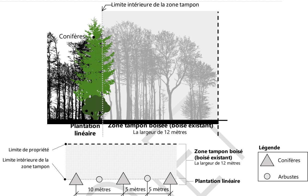
Figure 46 - Zone tampon constituée d'un boisé existant
