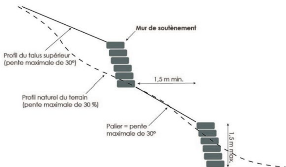
Figure 34 – Construction d'un mur de soutènement
