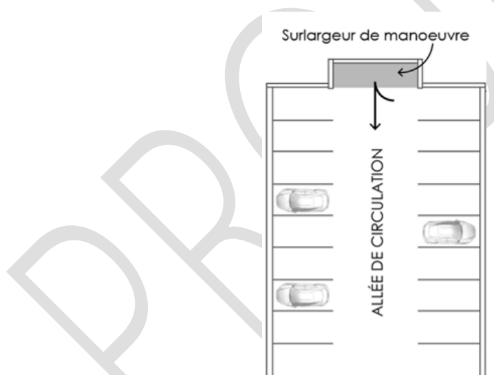
Figure 17 – Démonstration d'une surlargeur de manœuvre
