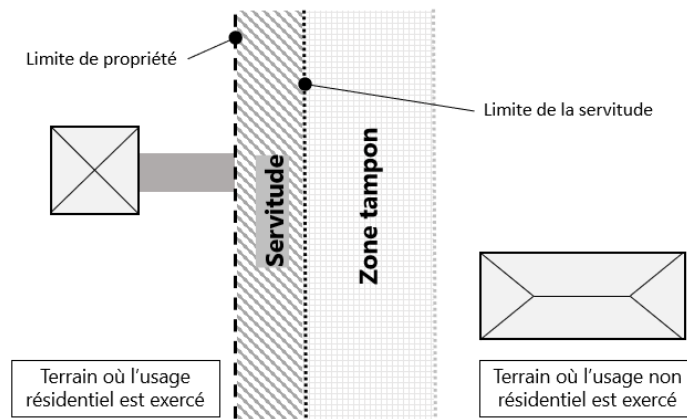
Figure 41 – Aménagement d'une zone tampon adjacente à une servitude
