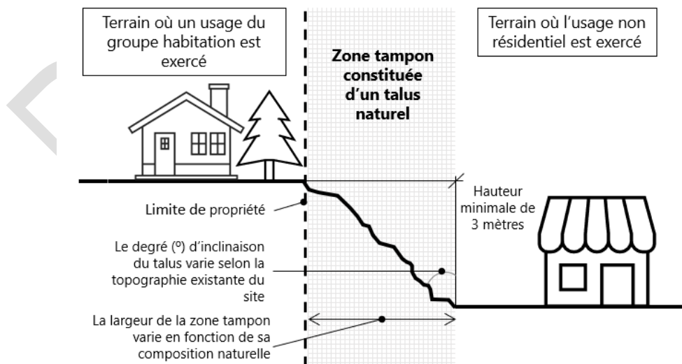
Figure 43 -Zone tampon constituée d'un talus naturel
