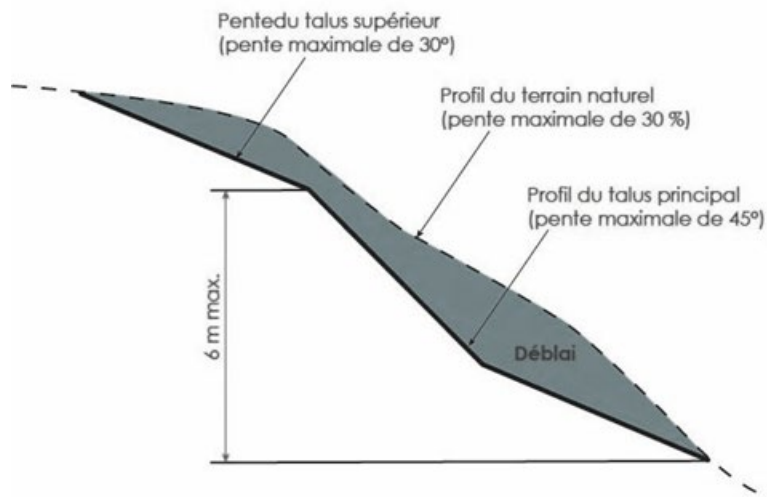
Figure 36 – Talus formé par des travaux de déblai
