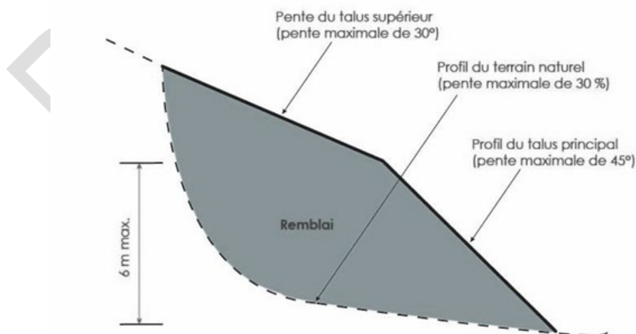
Figure 35 – Talus formé par des travaux de remblai
