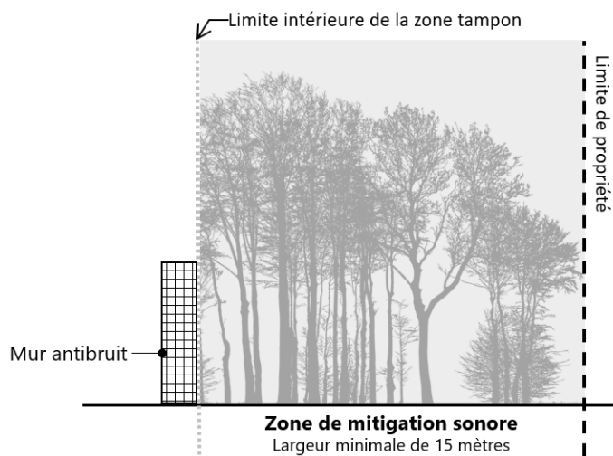
Figure 49 - Zone de mitigation sonore constituée d'un boisé existant et d'un mur antibruit
