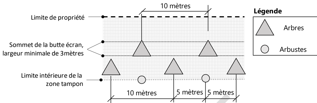
Figure 47 - Zone tampon constituée d'une butte-écran
