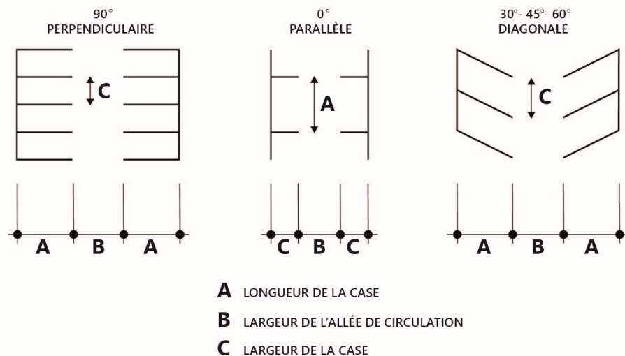
Figure 16 – Démonstration des dimensions des cases de stationnement
