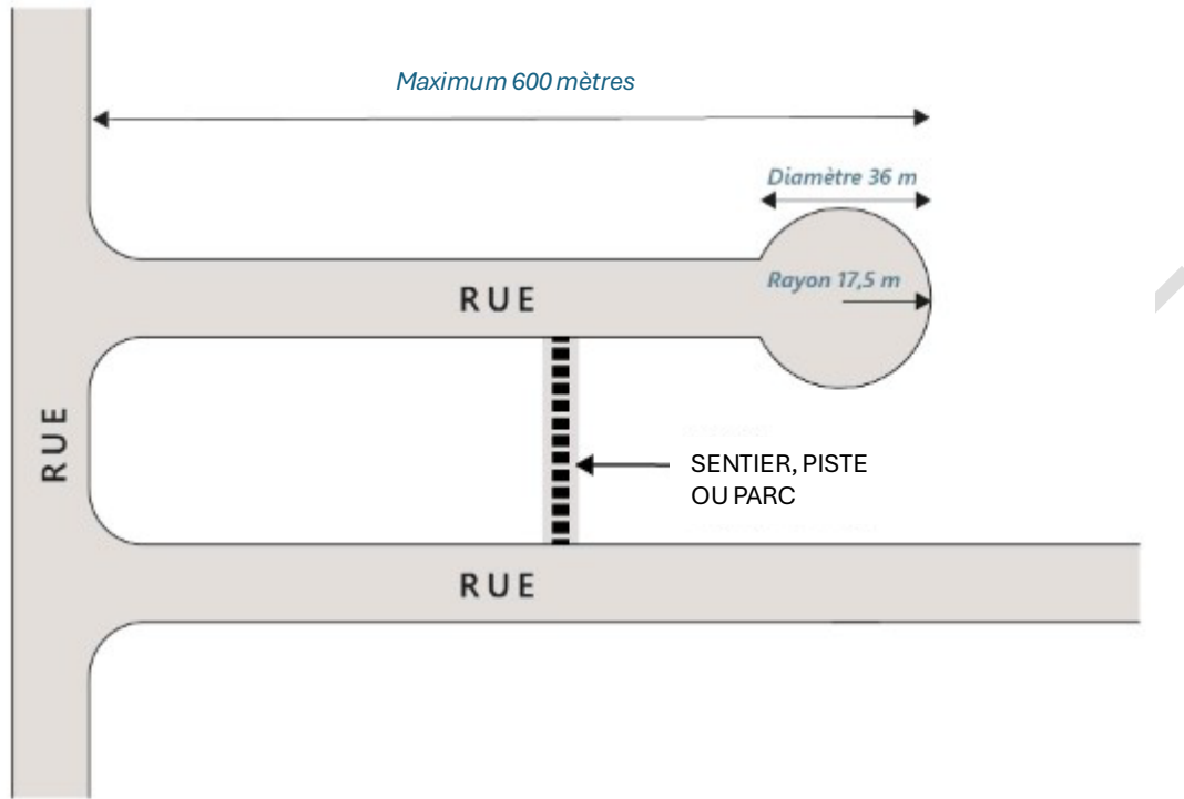
Figure 6 – Rue en cul-de-sac avec un sentier ou piste
