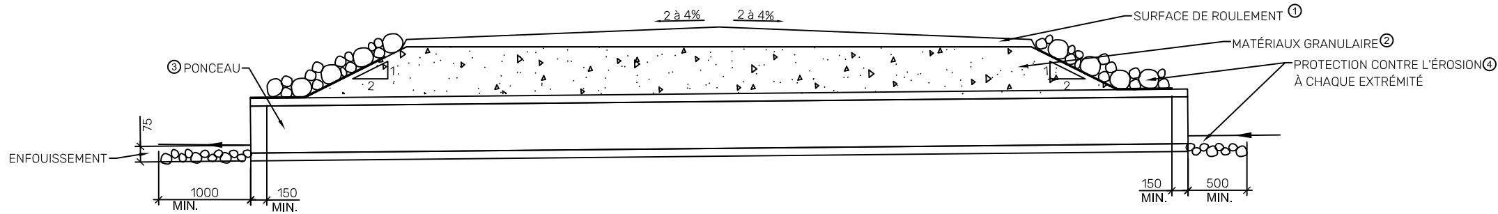
A PROFIL TYPE D'UNE ENTRÉE RÉSIDENTIELLE EN MILIEU RURAL
