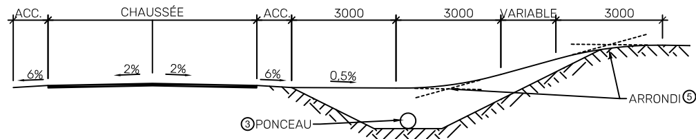
C PROFIL EN LONG EN DÉBLAI
